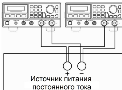
Рисунок 3-4. Параллельное подключение двух электронных нагрузок
